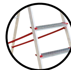
Tiras de refuerzo en 5, 6, 7 y 8 peldaños.
